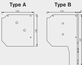
Zijkappen Carre 110
