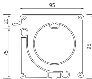
CARRE 95 Recht
