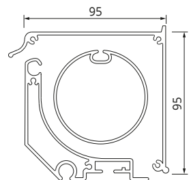
CARRE 95 Schuin
