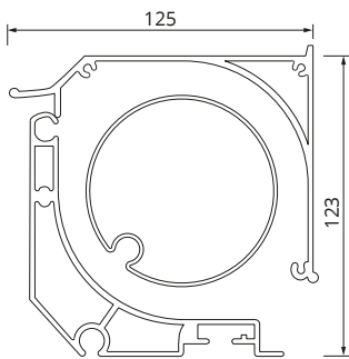
CARRE 110 Schuin
