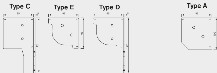
Zijkappen Carre 95
